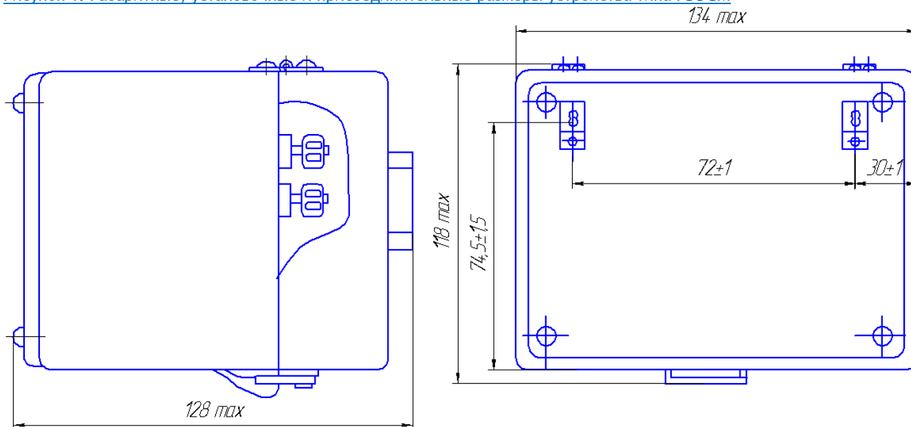
Рисунок 1 – Габаритные, установочные и присоединительные размеры устройства типа УСЗ ЗМ Размеры без предельных отклонений справочные
